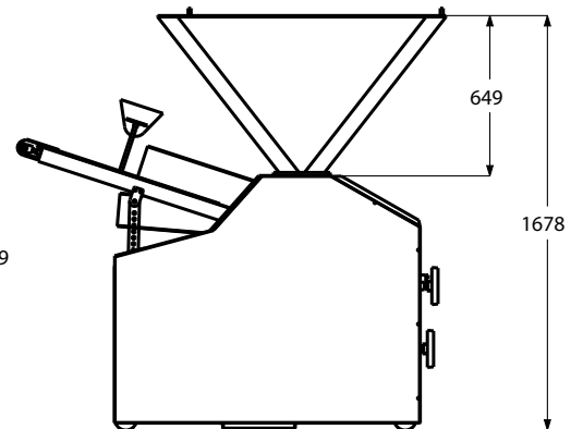
HOPPER 80L
