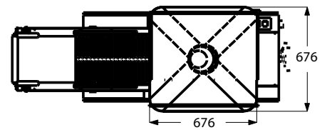
HOPPER 80L
