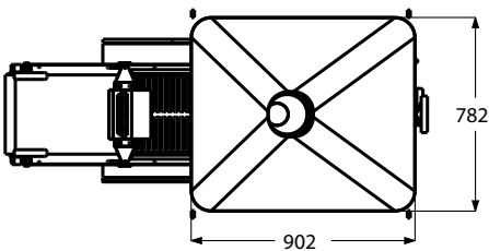
HOPPER 150L
